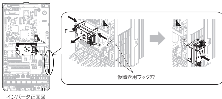
図 14 LED ステータスリング基板の取り外し
