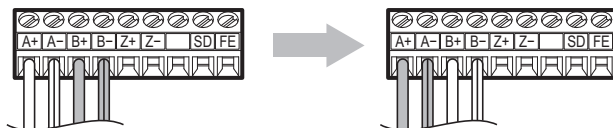
図 20 A 相と B 相の入れ替え
