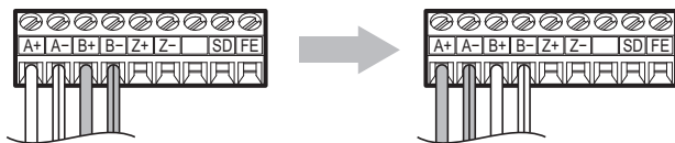
図 11 A 相と B 相の入れ替え
