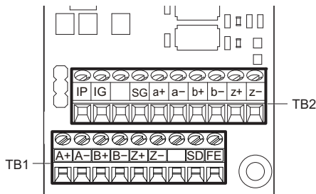
図 1 PG-X3 の各部の名称
