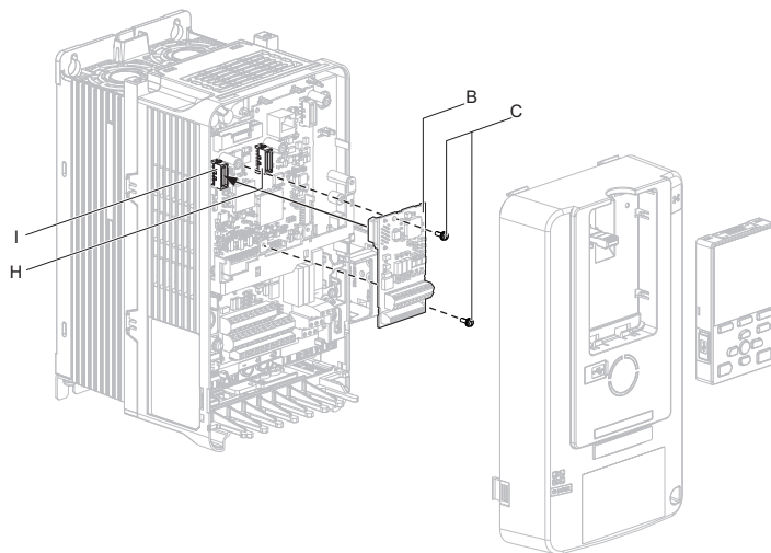
図 15 オプションカードの取付け
