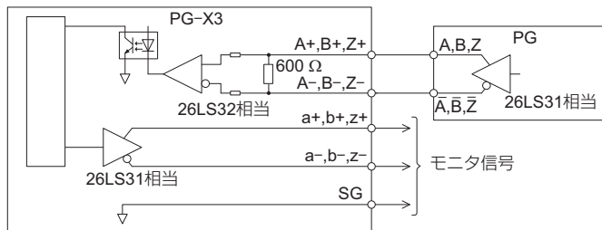
図 22 インタフェース回路図
