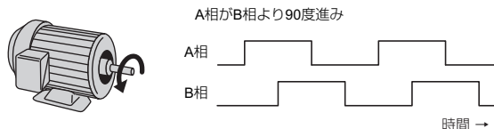
図 19 A 相, B 相信号位相関係図
