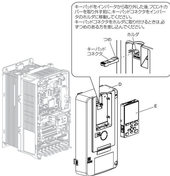
図 13 キーパッドとフロントカバーの取り外し
