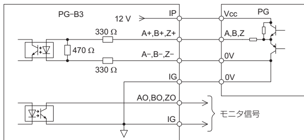
図 23 インタフェース回路図 (コンプリメンタリ型)
