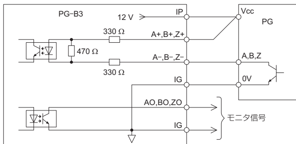
図 24 インタフェース回路図（オープンコレクタ型）
