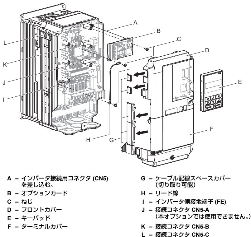
図 2 各部の名称 (例：CIMR-AA2A□)
