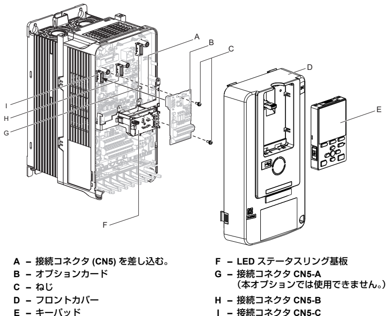
図 12 各部の名称
