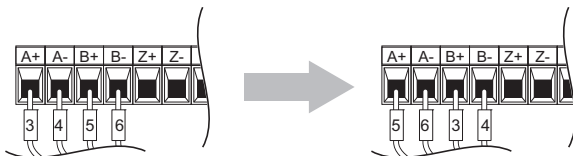
図 20 A 相と B 相の入れ替え
