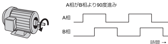
図 19 A 相、B 相信号位相関係図
