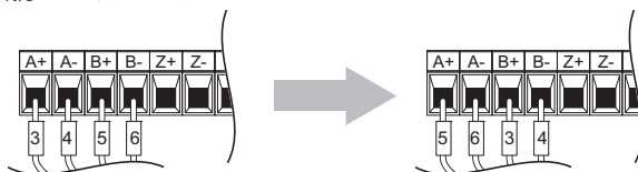
図 11 A 相と B 相の入れ替え
