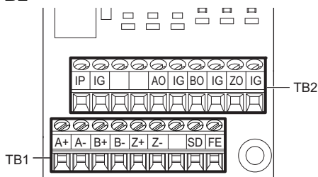
図 1 PG-B3 の各部の名称
