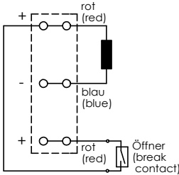
Schaltbild: (circuit diagram)
